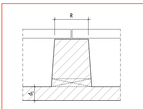
Detail-D
